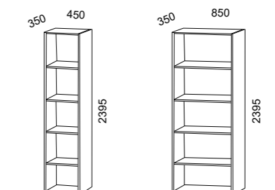
Estanterías H=2395 / Rayonnages H=2395
